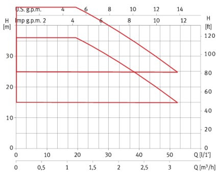
KENNLINIE 0920048M
