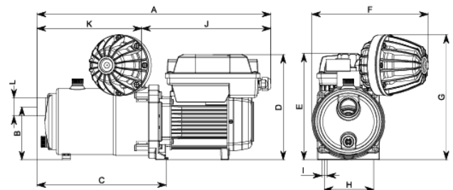
MASSZEICHNUNG 0920048M
