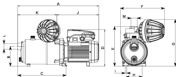
MASSZEICHNUNG 0920047M
