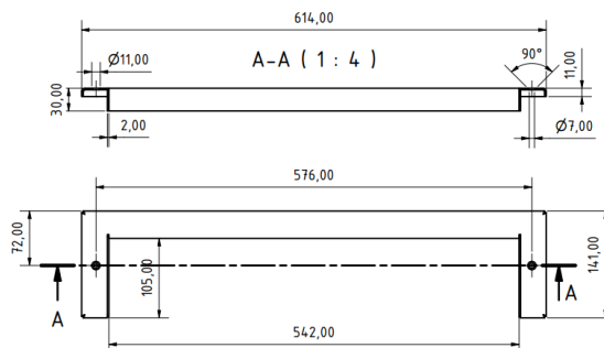
MASSZEICHNUNG: 0010017
