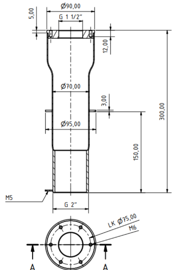
MASSZEICHNUNG: 0010019
