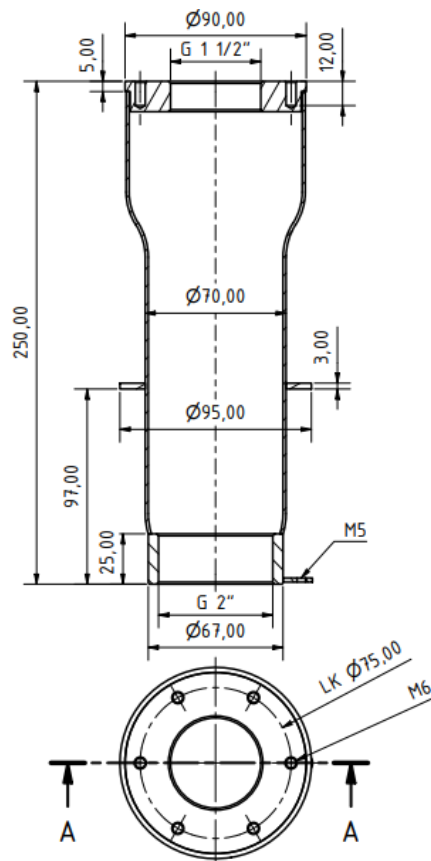
MASSZEICHNUNG: 0010018
