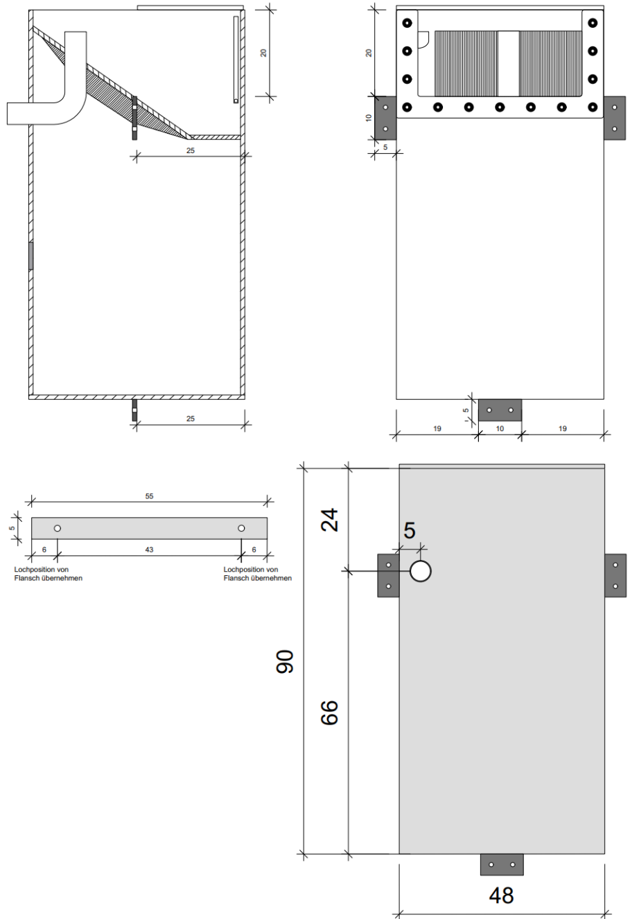
MASSZEICHNUNG:
